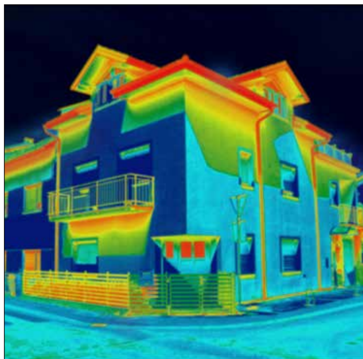
Ein Wärmedämm-Verbundsystem braucht angepasste Detaillösungen, damit sich Fenster, Türen und Balkone ohne Wärmebrücken in die Dämmschicht integrieren lassen
